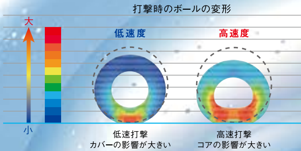
中空3ピース構造による効果 ※グラフは、アシックススポーツ工学研究所の実験データより ●ティーショットの高速打撃では、ハードな打撃感に。 ●グリーン周りの低速打撃では、ソフトな打撃感に。
