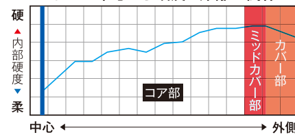
ボール中心から硬度と距離の関係
